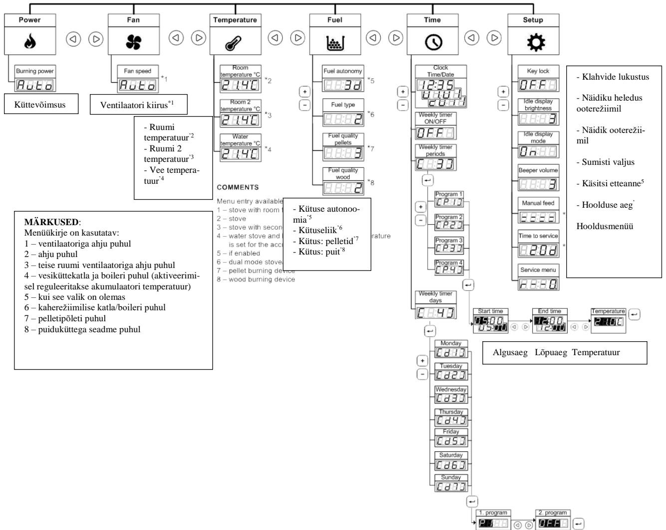
Joonis 25: Menüüstruktuur
